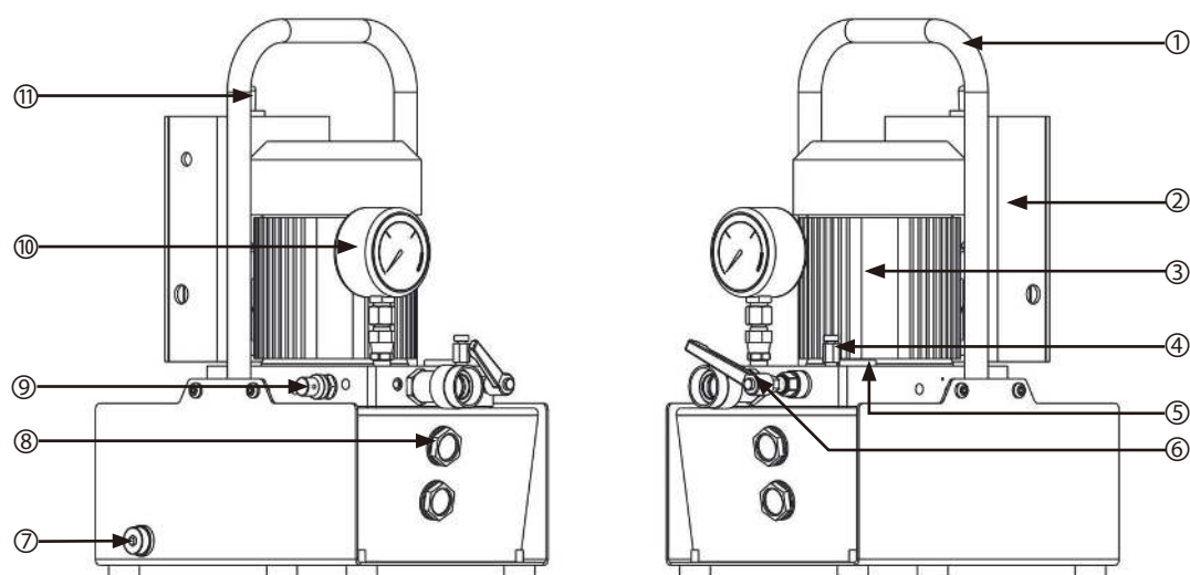
▼ HC3MV43 产品示意图:
