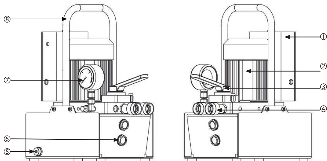
▼ HC3EV 产品示意图:
