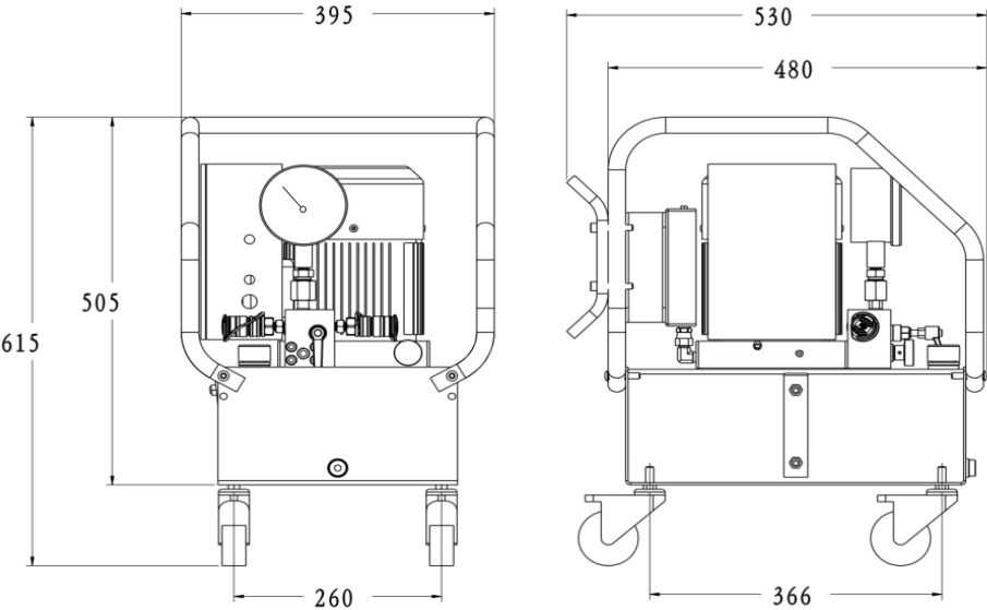
▼ EPW-F20 外形尺寸图:
