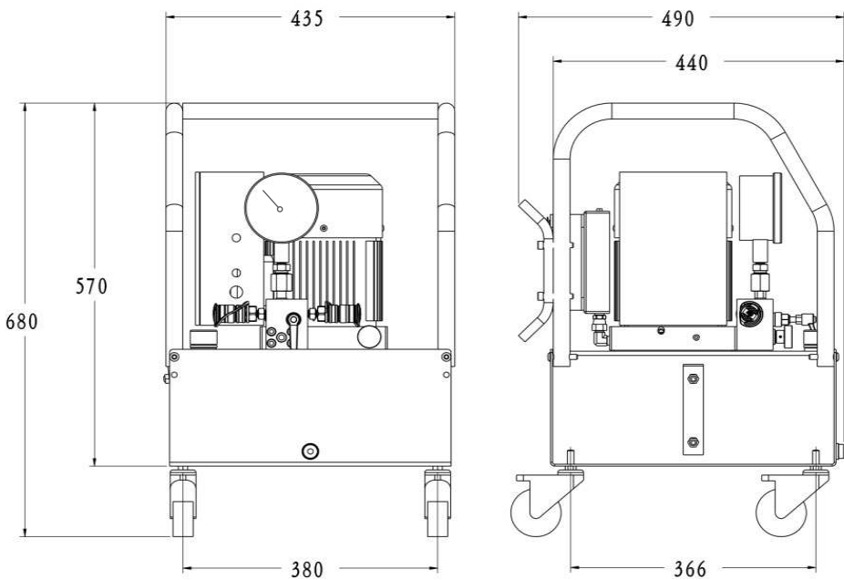
▼ EPW-F20 外形尺寸图:
